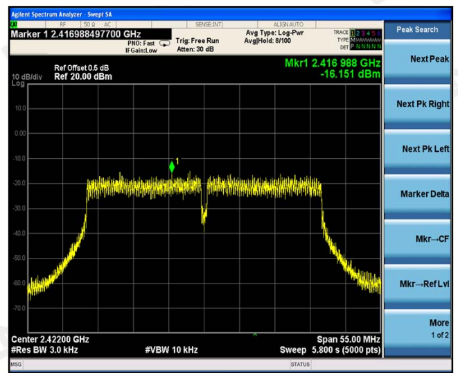
802.11n(HT40)
