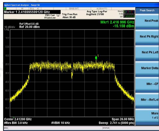
802.11n(HT20)
