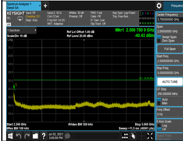
802.11n(HT40),2452MHz,Ant0,Plot 4,2500MHz~5000MHz
