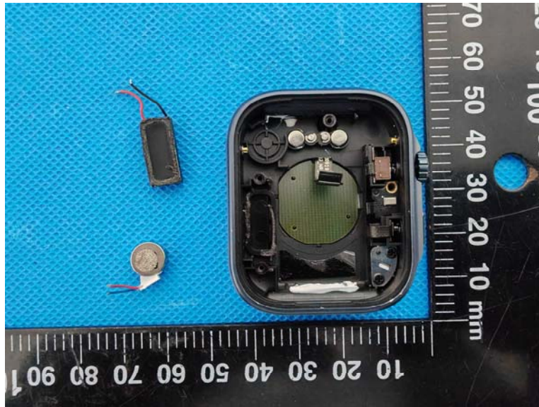
Motor 1
