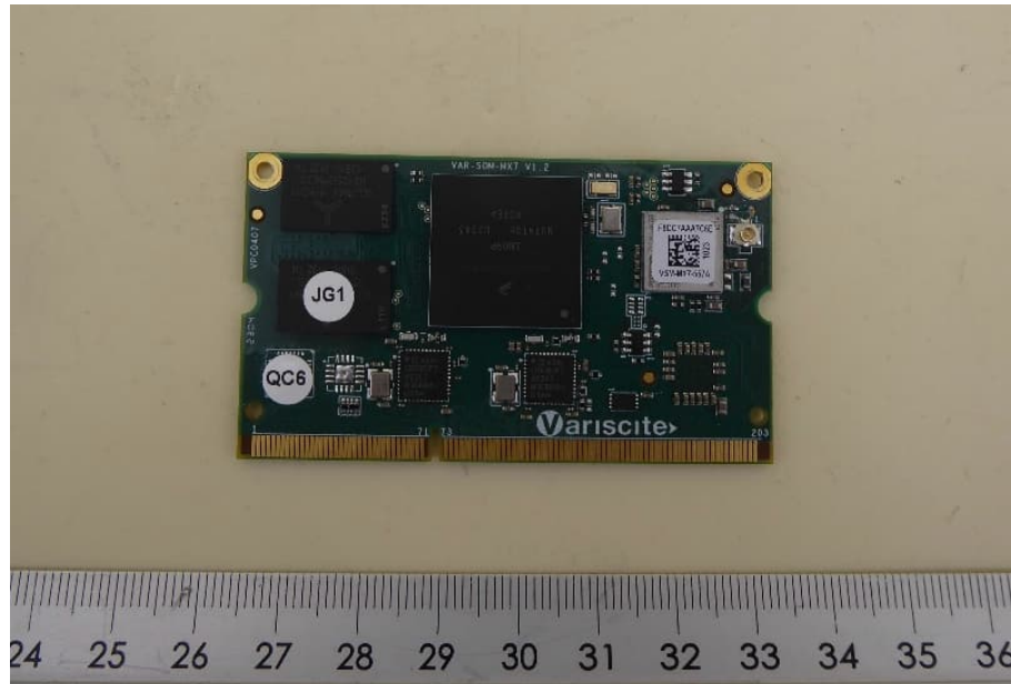
Variscite Module top view
