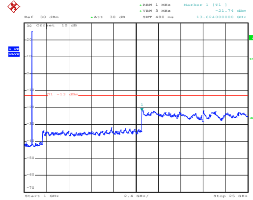
1GHz~25GHz
