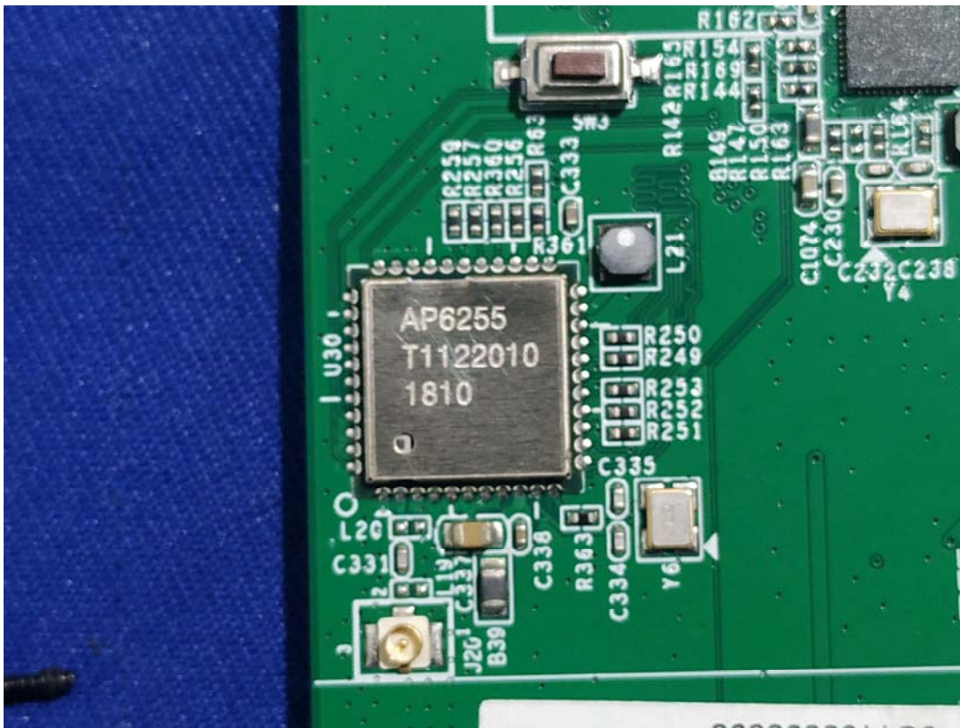
BT&WIFI Module
