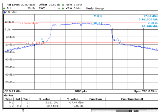
ac80_5210MHz_Chain 0
