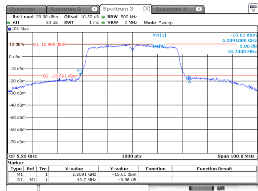
n40_5230MHz_Chain 0
