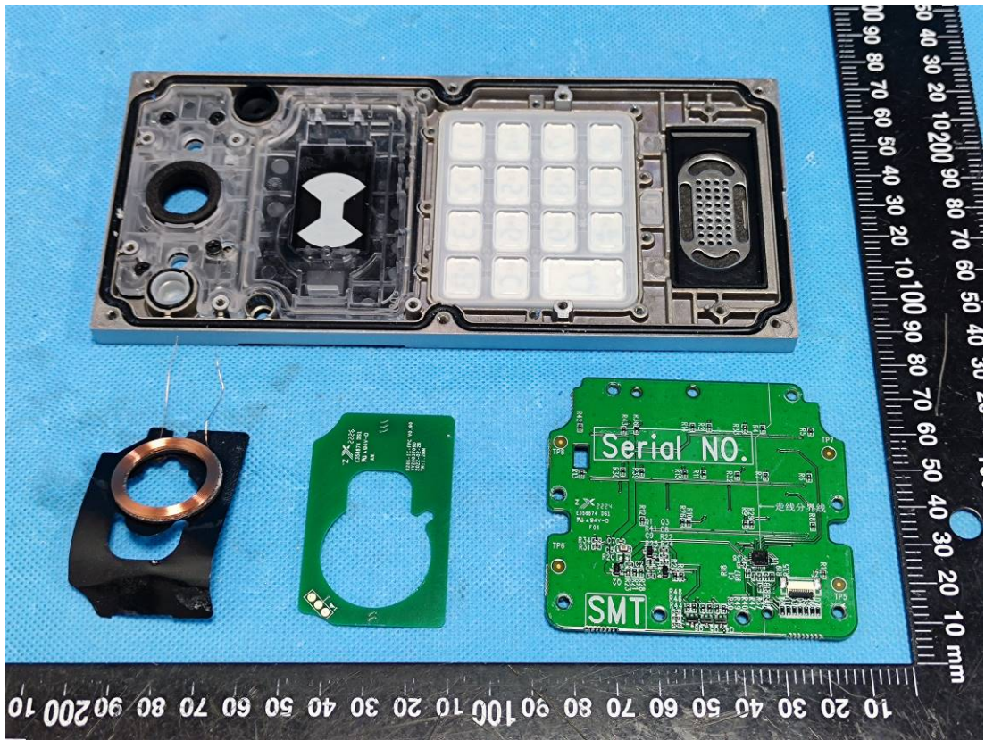
RFID Antenna
