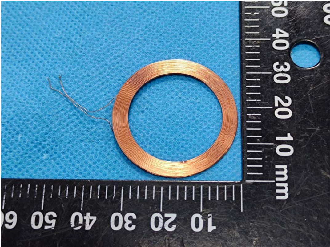
RFID Antenna
