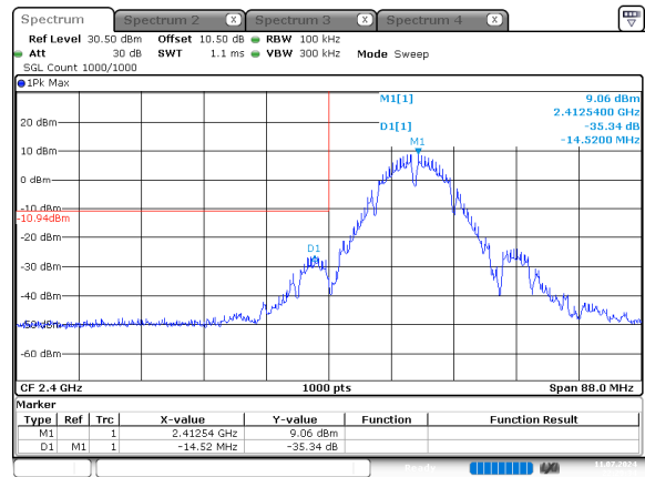
b_2412MHz_Chain 0
