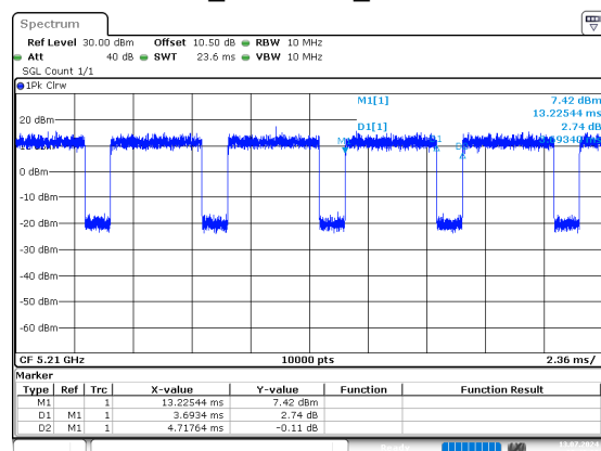
ac80_5210MHz_Chain 0
