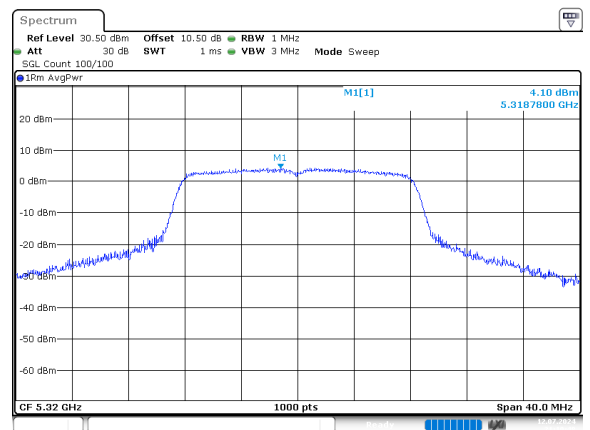
a_5320MHz_Chain 0
