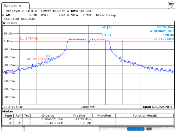
a_5720MHz_Chain 0
