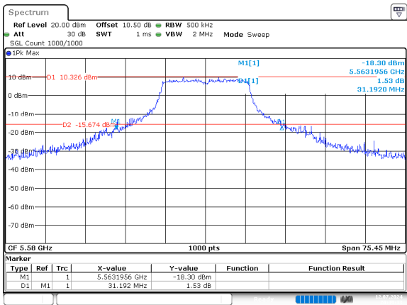
a_5580MHz_Chain 0
