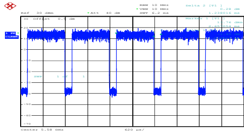
a_5580MHz_Chain 0
