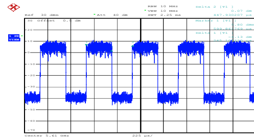
ac80_5610MHz_Chain 0
