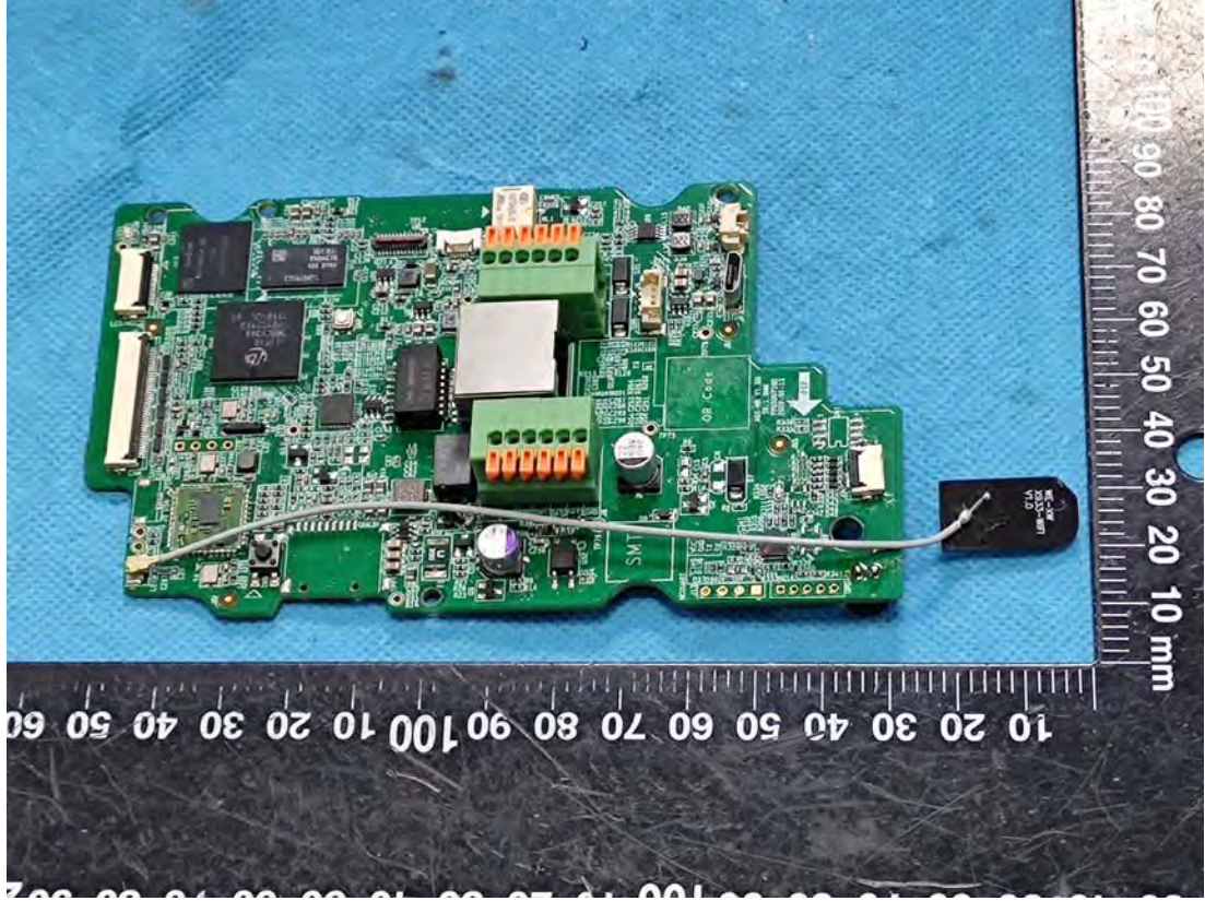
BLE Antenna
