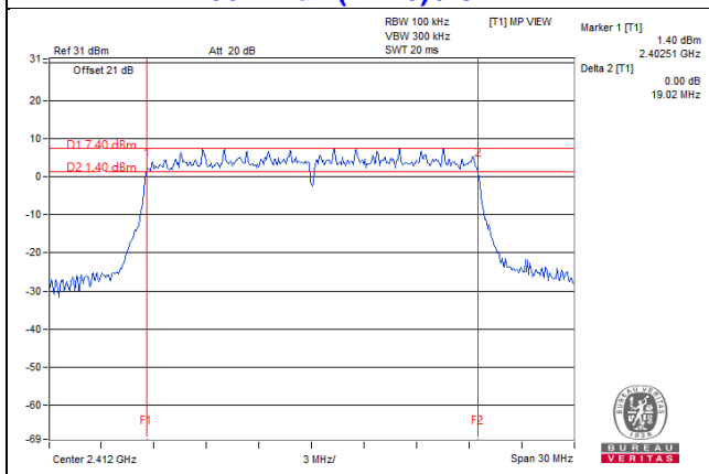
802.11ax (HE20) / CH1
