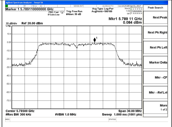
802.11n20-5785MHz
