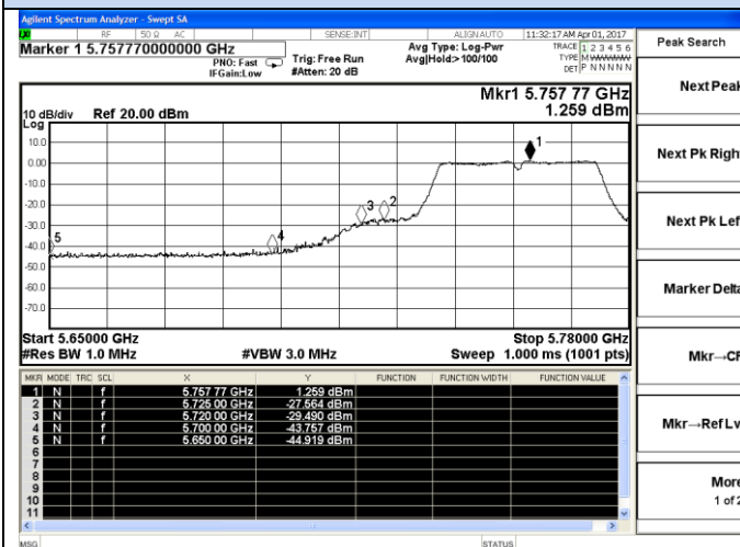
802.11n40-5755MHz-Lower
