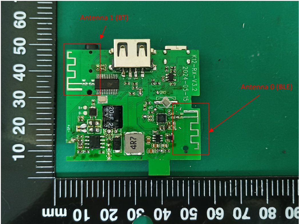
Antenna
