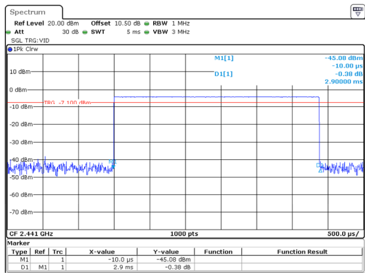
GFSK_Hopping_DH5 2.900ms
