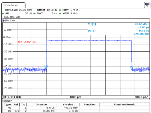
\pi/4 -DQPSK_Hopping_2DH5 2.905ms
