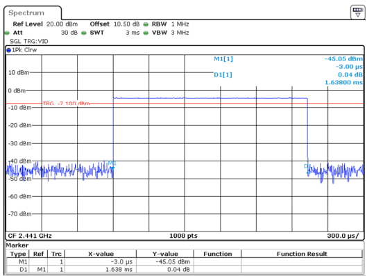
GFSK_Hopping_DH3 1.638ms
