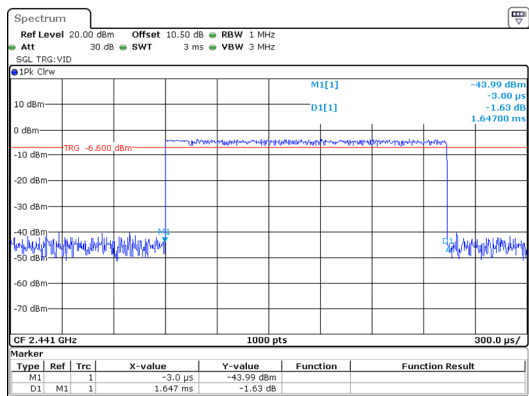
\pi/4 -DQPSK_Hopping_2DH3 1.647ms
