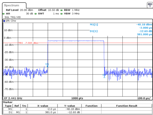
GFSK_Hopping_DH1 0.381ms
