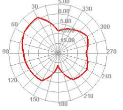
2450.000MHz E2
