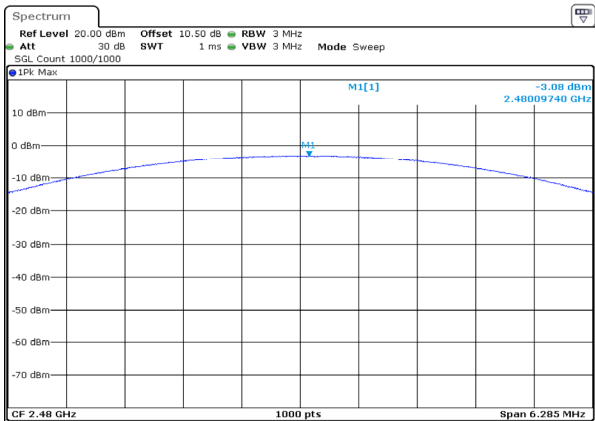
\pi/4 -DQPSK_High -3.08dBm
