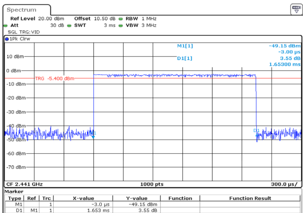
\pi/4 -DQPSK_Hopping_2DH3 1.653ms
