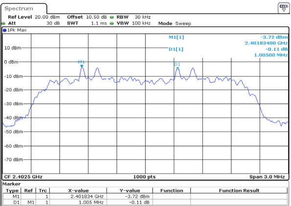
\pi/4 -DQPSK_Low 1.005MHz
