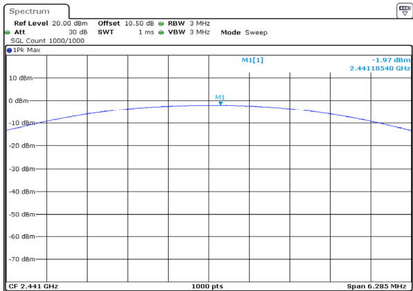
\pi/4 -DQPSK_Middle -1.97dBm
