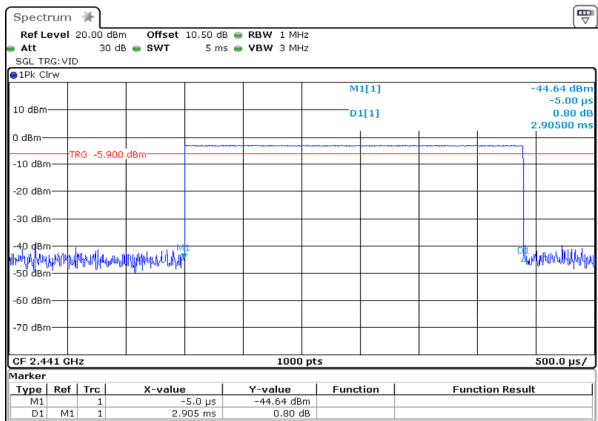
GFSK_Hopping_DH5 2.905ms
