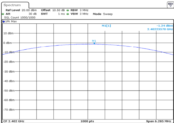
\pi/4 -DQPSK_Low -1.24dBm
