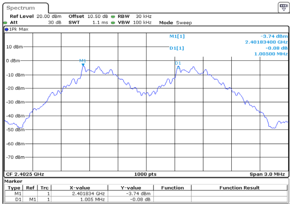
GFSK_Low 1.005MHz
