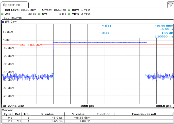
GFSK_Hopping_DH3 1.650ms
