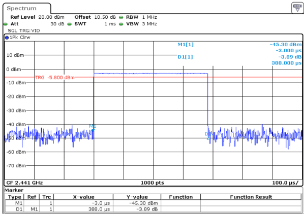
GFSK_Hopping_DH1 0.388ms
