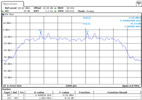
\pi/4 -DQPSK_Middle 1.005MHz
