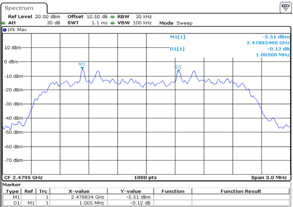
\pi/4 -DQPSK_High 1.005MHz
