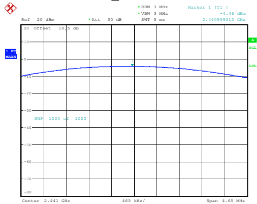
GFSK_Middle -4.46dBm
