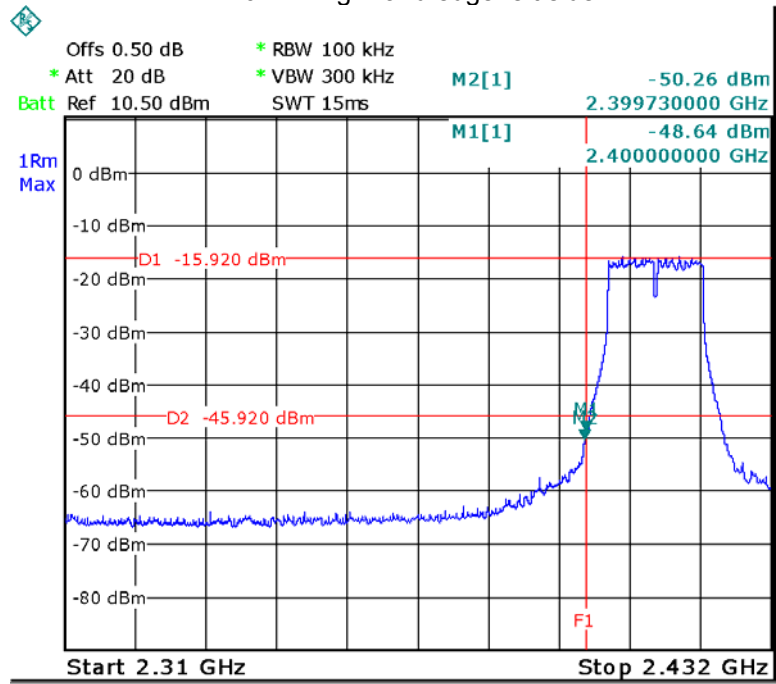
ANT0 TX 11g: Band edge-left side
