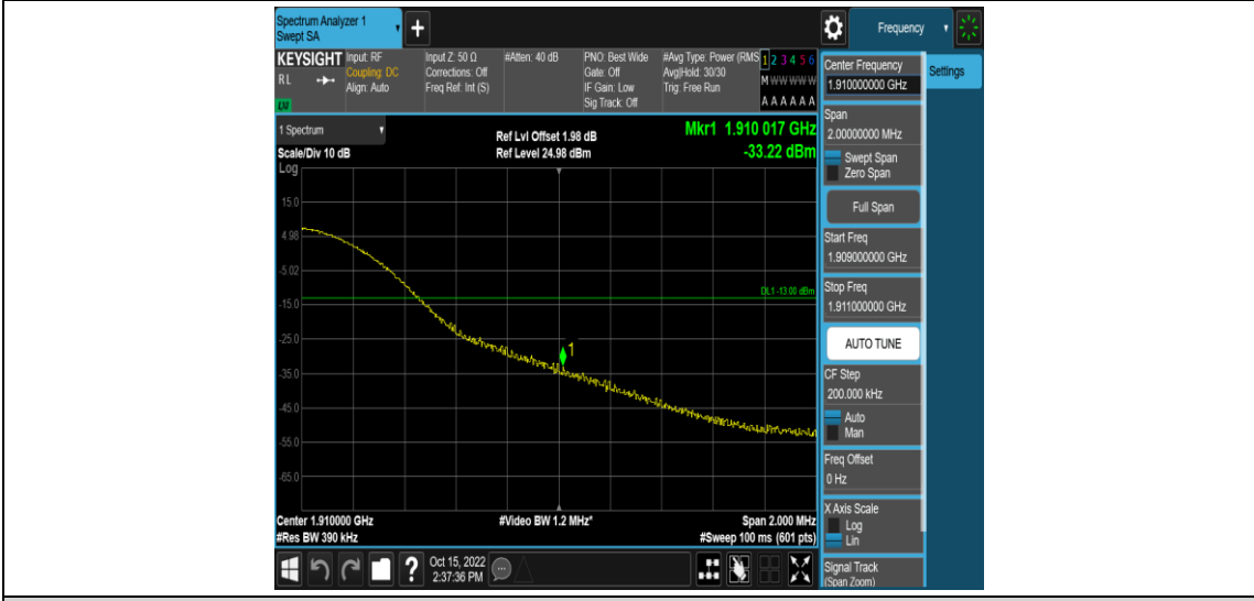
Band2-20MHz-16QAM-19100-100RB#0
