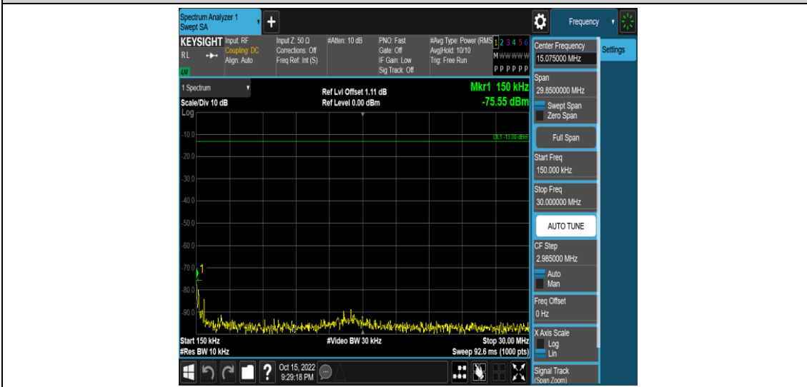
Band66-20MHz-QPSK-132572-1RB#0-Range3:30~1000MHz
