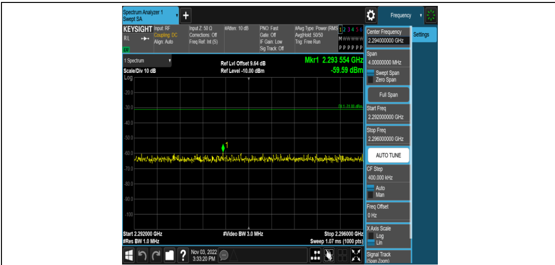
Band40-5MHz-QPSK-39200-1RB#0-Range7:2296~2300MHz
