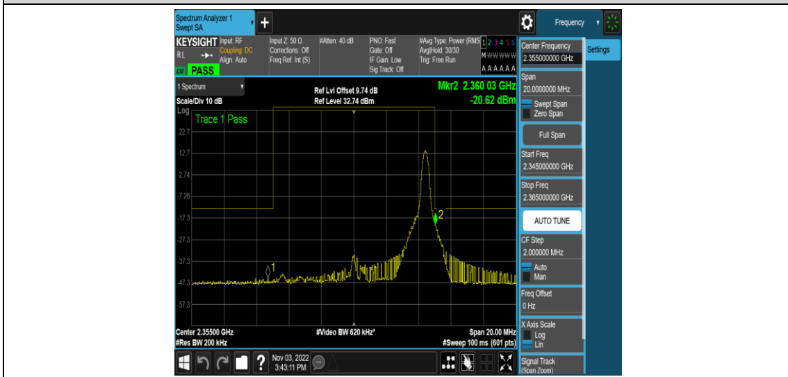
Band40-10MHz-QPSK-39200-50RB#0
