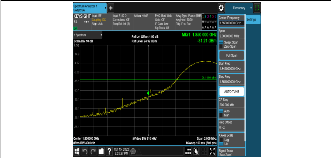
Band2-15MHz-16QAM-18675-1RB#74
