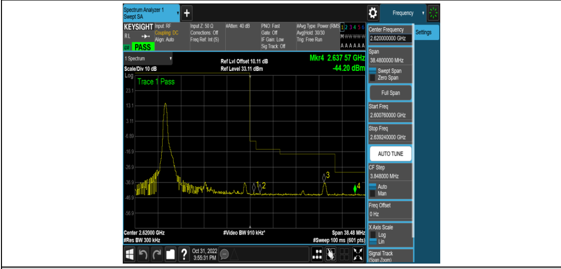
Band38-15MHz-QPSK-38175-1RB#74
