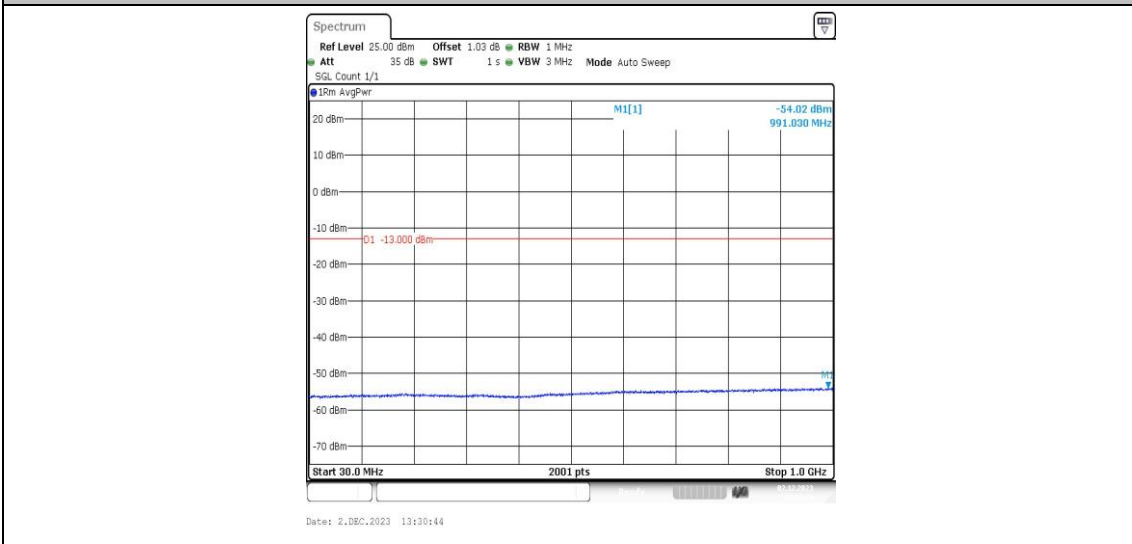
Band2-9538-1-30~1000MHz-PASS
