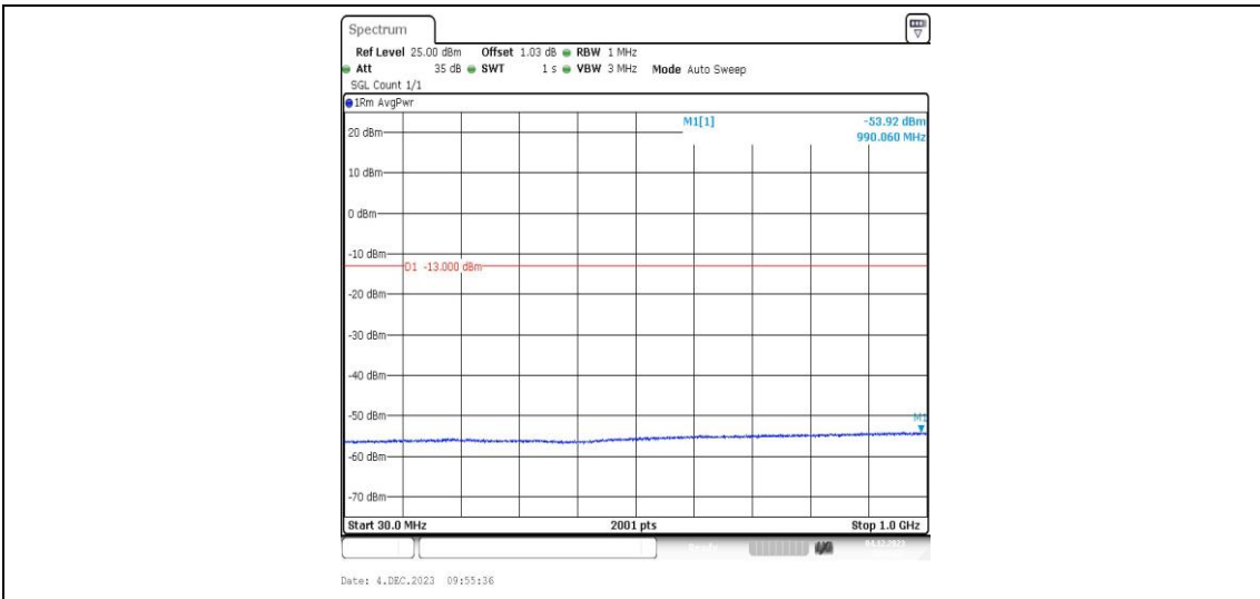
Band4-1413-4-30~1000MHz-PASS
