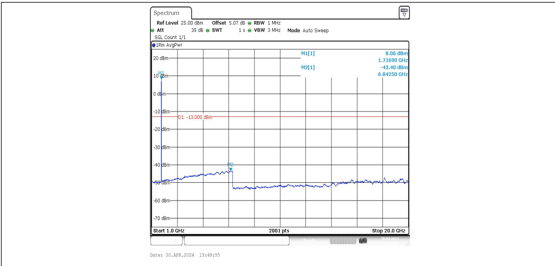
Band4-1312-1-1000~20000MHz-PASS
