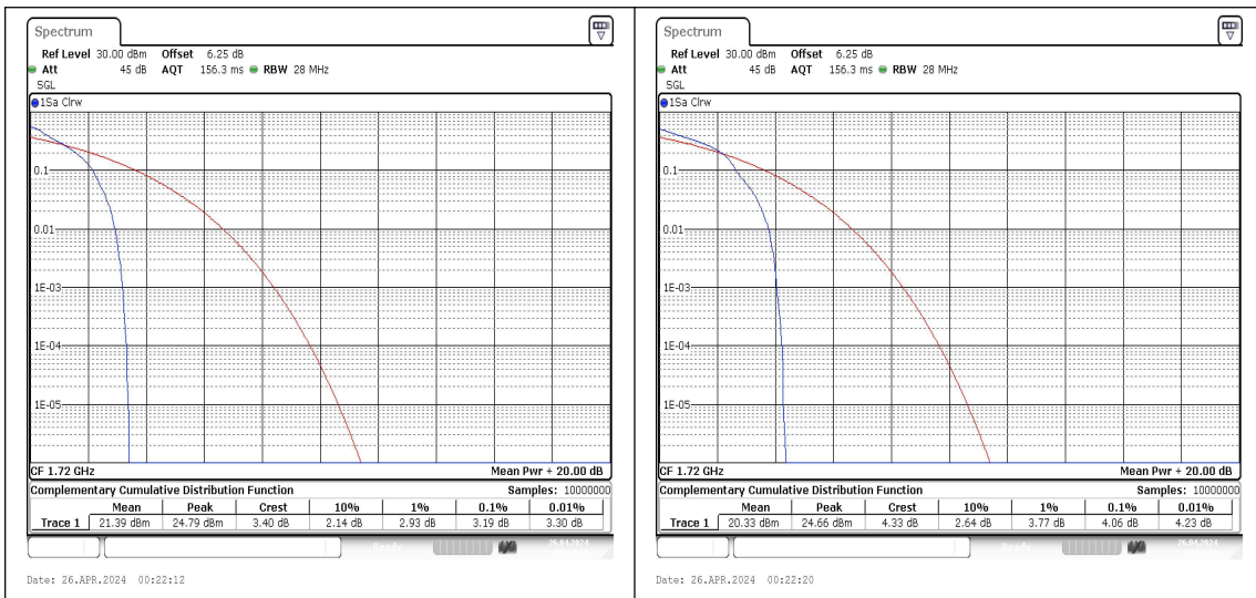
Band66-20MHz-QPSK-132072-1RB#0-PASS Band66-20MHz-16QAM-132072-1RB#0-PASS
