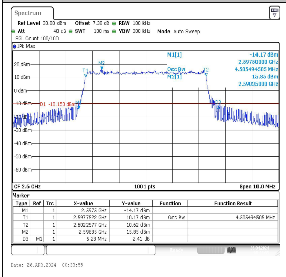
41(2555-2655)-5MHz-QPSK-40690-25RB#0-PAS S
