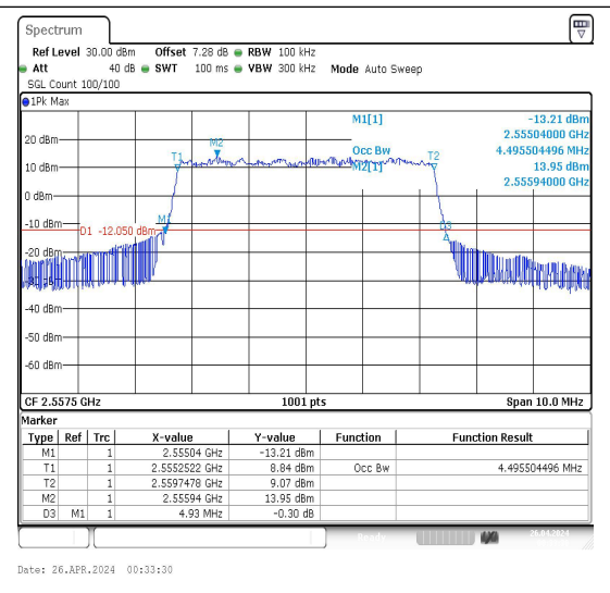
41(2555-2655)-5MHz-16QAM-40265-25RB#0-PAS S
