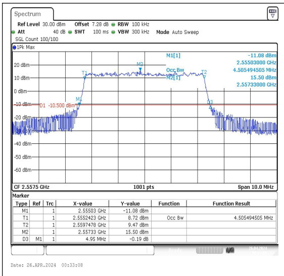
41(2555-2655)-5MHz-QPSK-40265-25RB#0-PAS S
