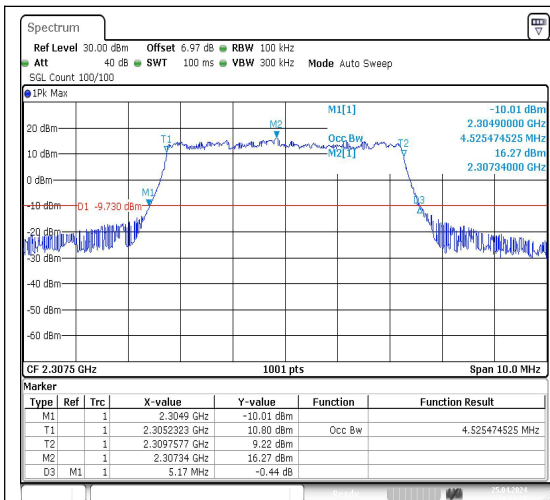
40(2305-2315)-5MHz-QPSK-38725-25RB#0-PAS
