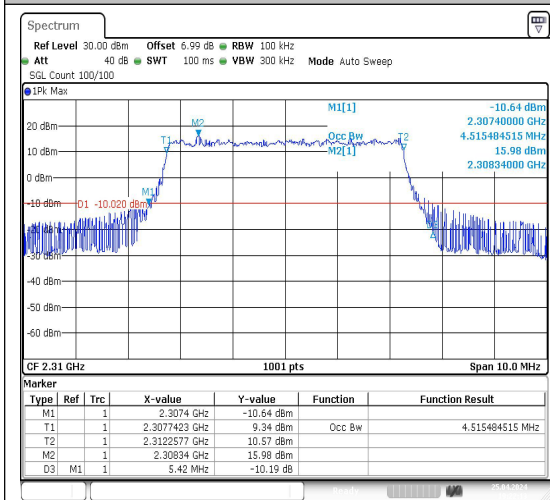
40(2305-2315)-5MHz-QPSK-38750-25RB#0-PAS
