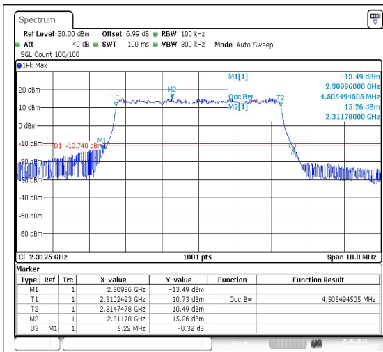
40(2305-2315)-5MHz-QPSK-38775-25RB#0-PAS S
