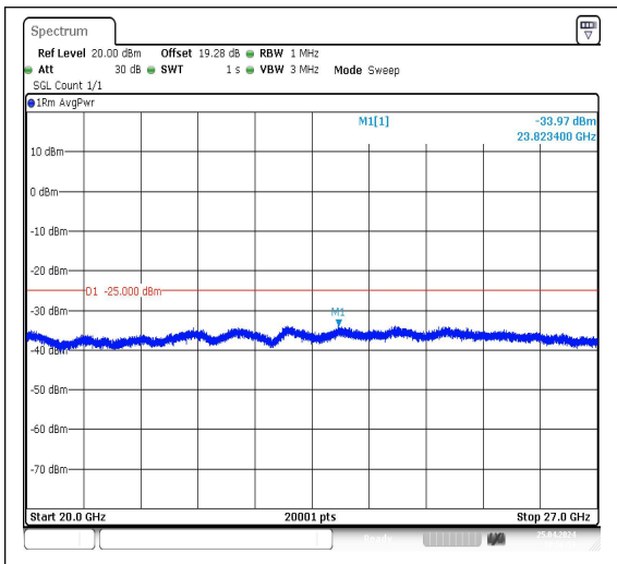
Band7_20MHz_QPSK_20850_1RB#0_20000~27000_000_20000~27000
