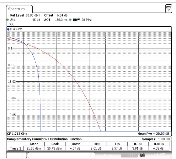
Band4-10MHz-QPSK-20000-1RB#0-PASS
