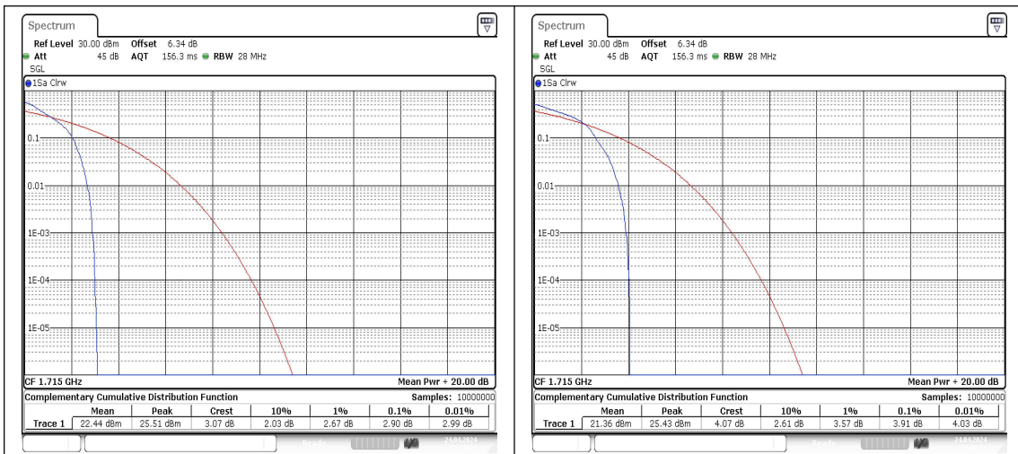
Band4-10MHz-QPSK-20000-1RB#0-PASS
