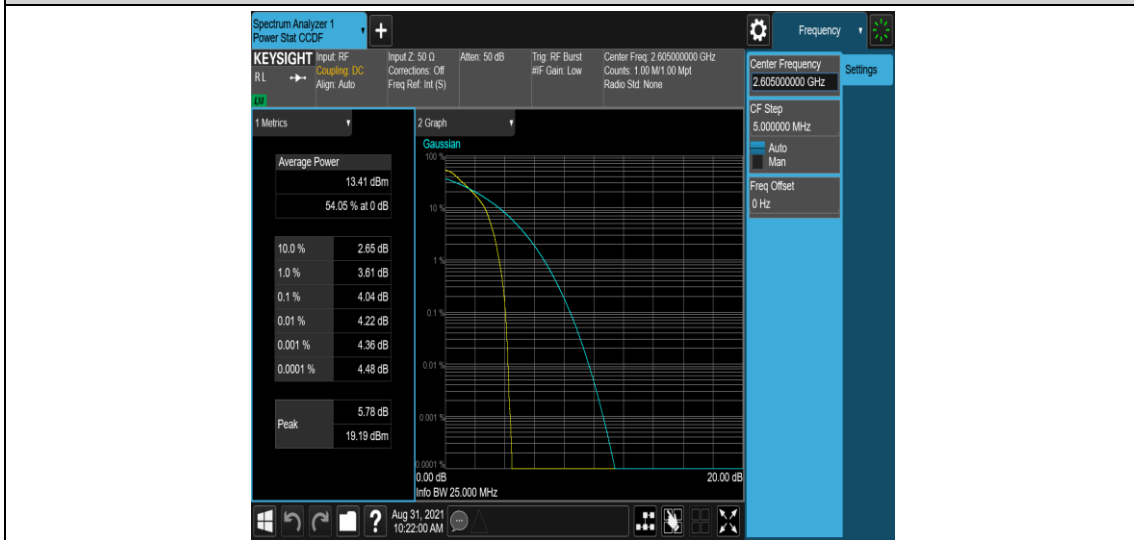
Band41-10MHz-QPSK-40740-50RB#0
