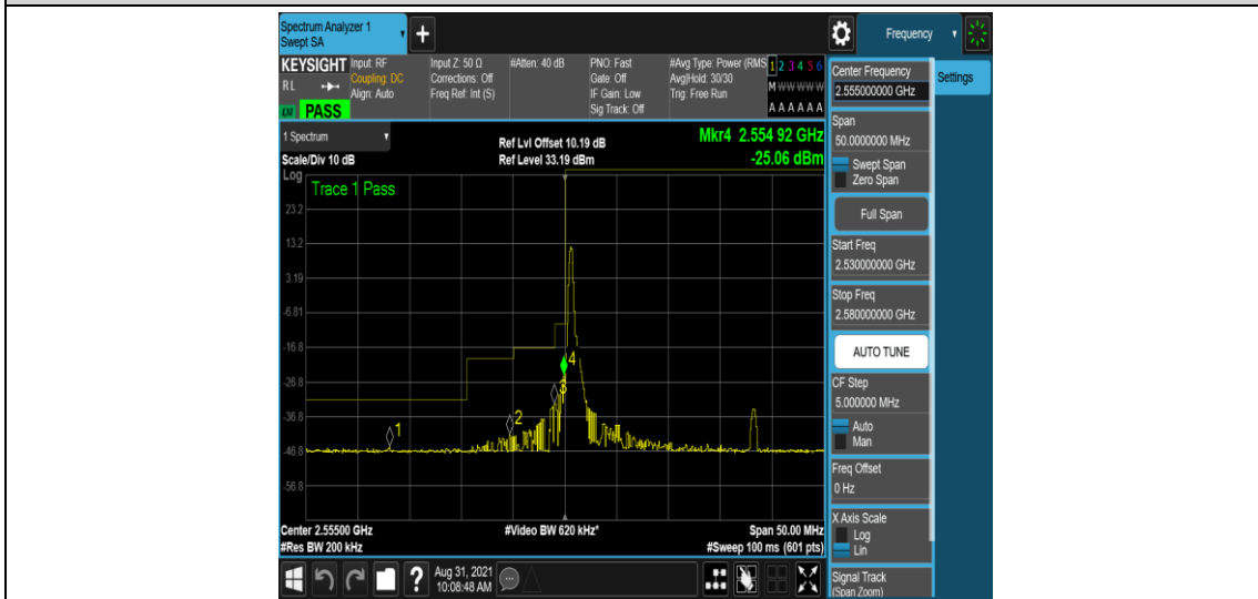
Band41-10MHz-QPSK-40290-1RB#0
