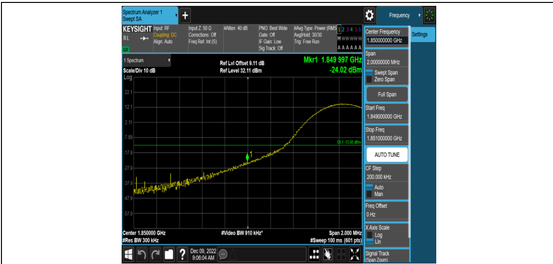
Band2-15MHz-16QAM-18675-1RB#74
