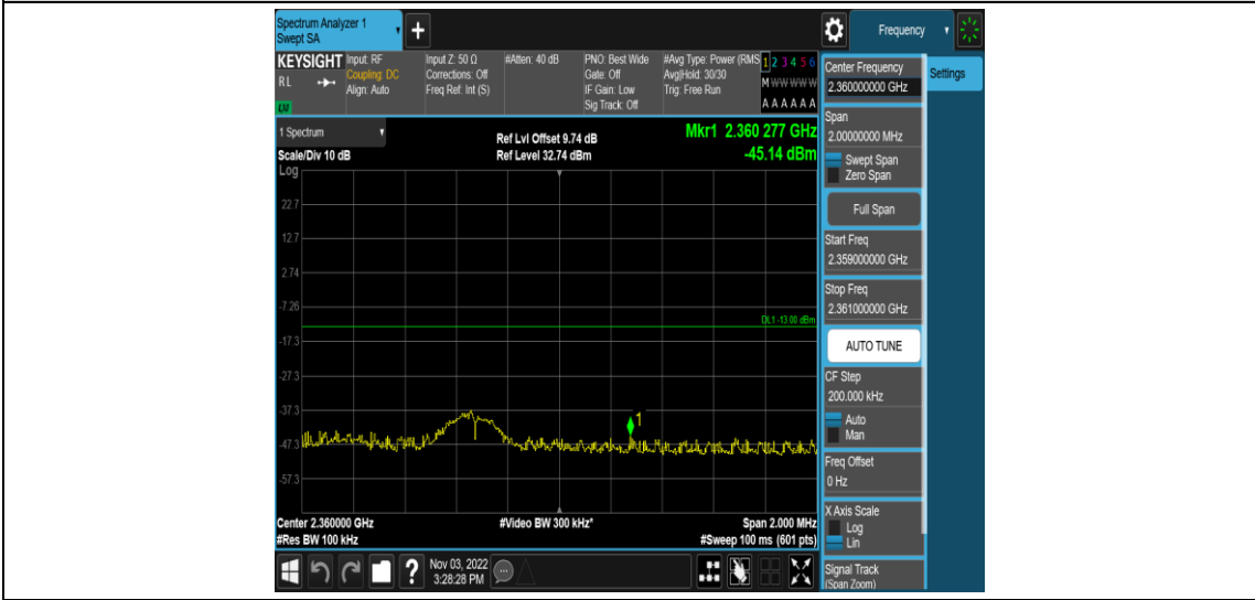
Band40-5MHz-QPSK-39225-1RB#24
