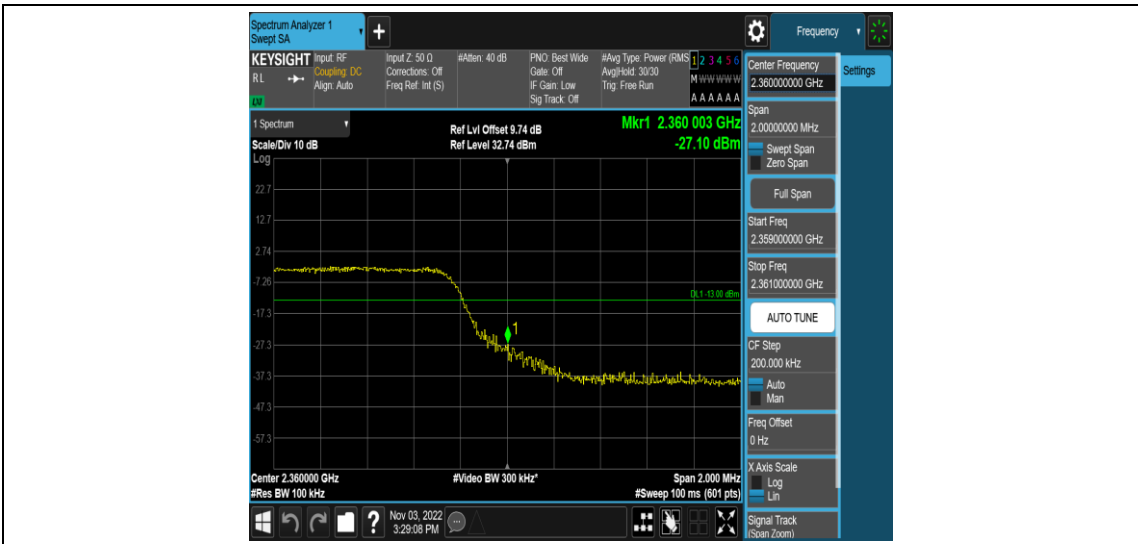
Band40-10MHz-QPSK-39200-1RB#0
