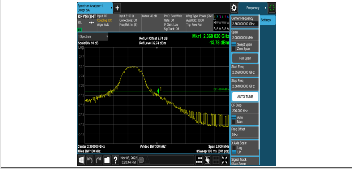
Band40-5MHz-QPSK-39225-25RB#0
