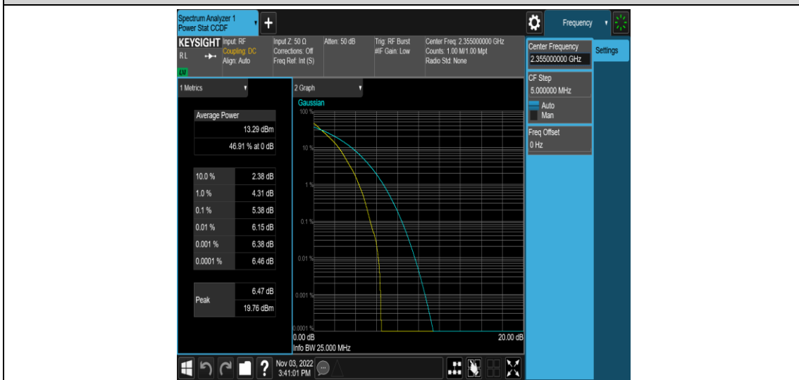
Band40-5MHz-QPSK-39225-1RB#0
