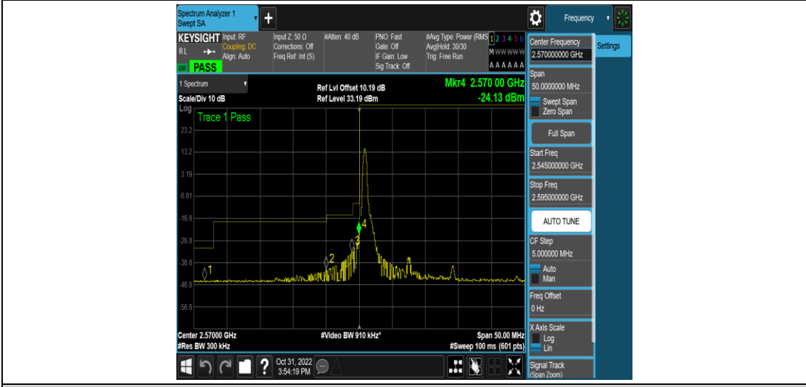
Band38-15MHz-QPSK-37825-1RB#74
