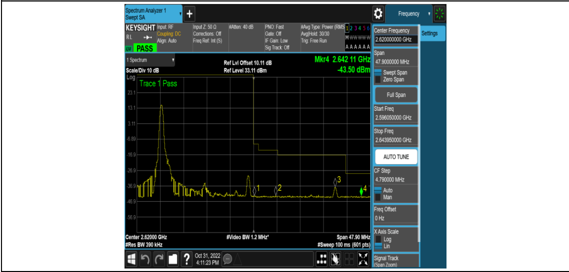
Band38-20MHz-QPSK-38150-1RB#99
