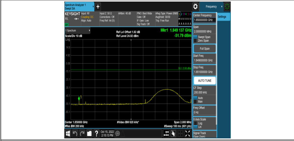
Band2-10MHz-QPSK-18650-50RB#0
