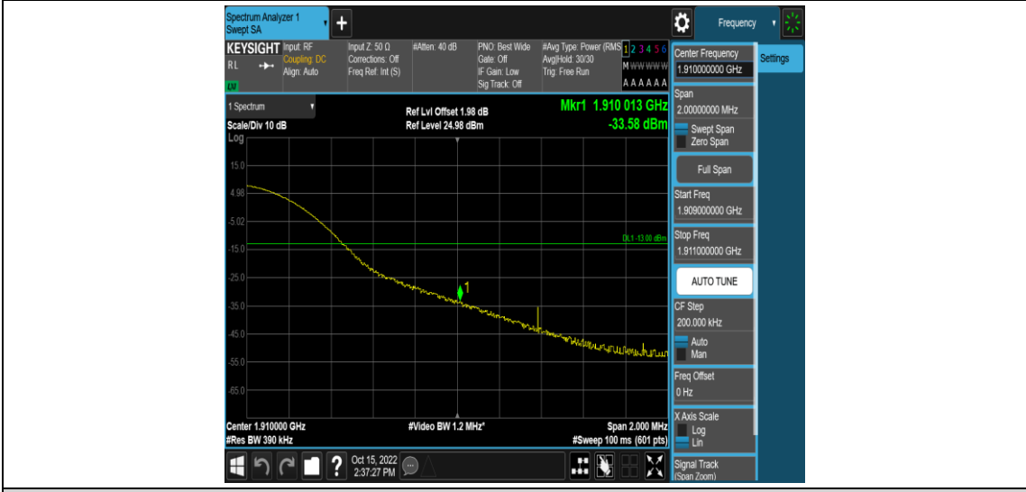
Band2-20MHz-QPSK-19100-100RB#0
