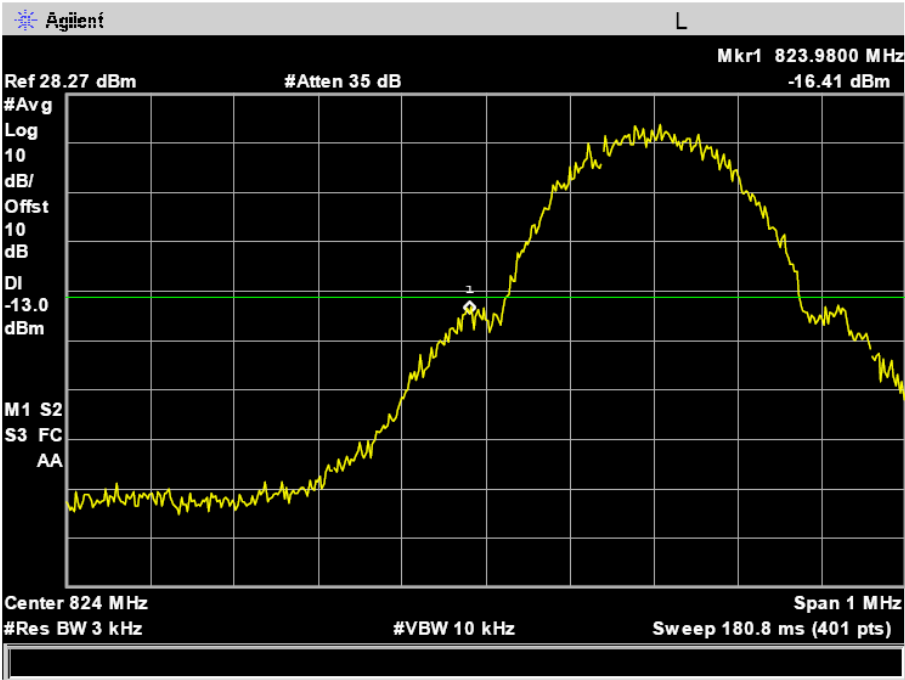
Low Band Edge EGPRS 850 BAND CH 128
