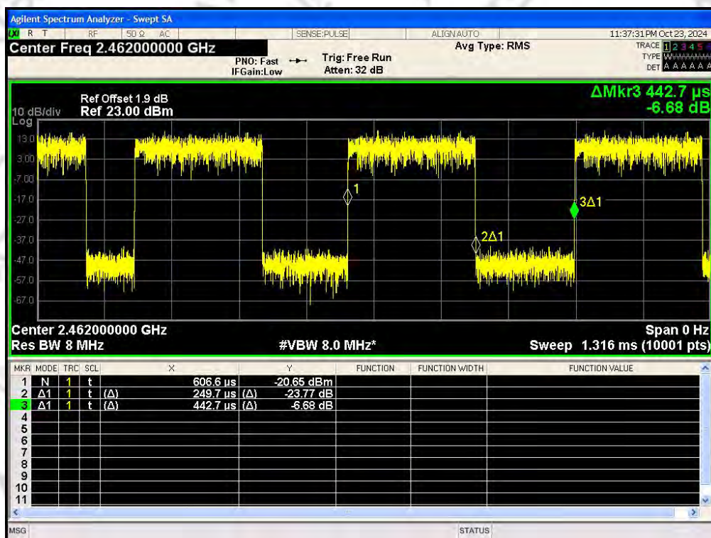
IEEE 802.11g_20MHz_Channel 11
