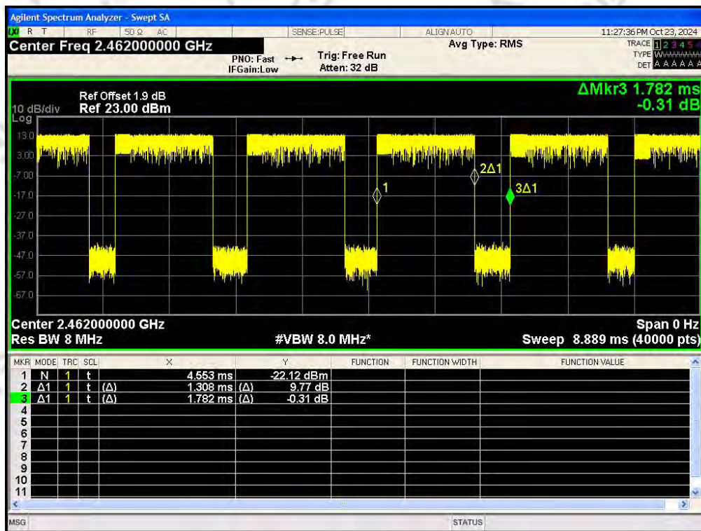
IEEE 802.11b_20MHz_Channel 11
