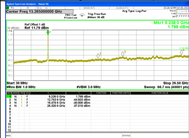
W52_11ac40_Higher_Band edge
