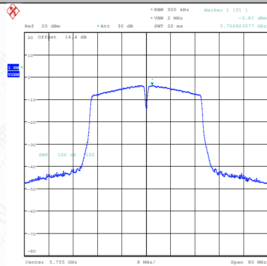
11N40SISO-Ant1-5755-PASS
