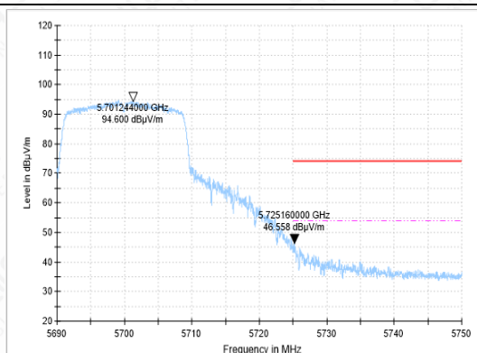
BANDEGE-11AC-CH140-AV
