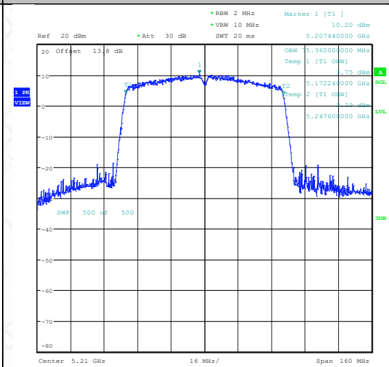
11AC80SISO-Ant1-5210
