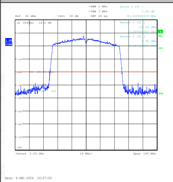
11AC80SISO-Ant1-5290
