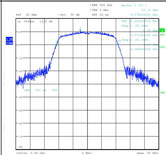
11A-Ant1-5580
