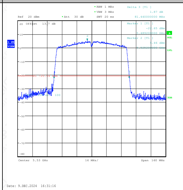
11AC80SISO-Ant1-5530
