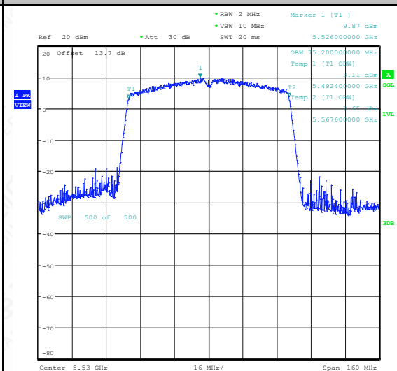
11AC80SISO-Ant1-5530
