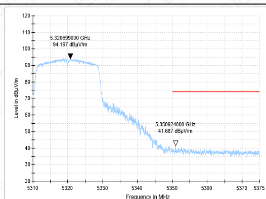
BANDEGE-11AC-CH64-AV
