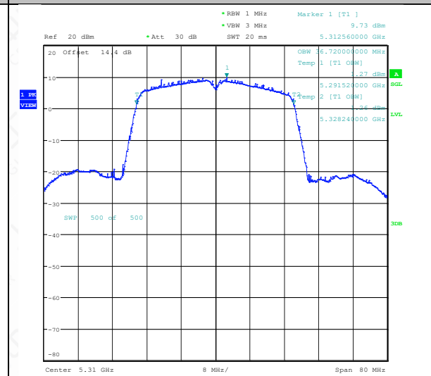
11N40SISO-Ant1-5310
