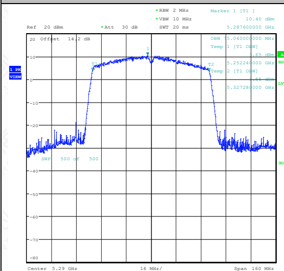
11AC80SISO-Ant1-5290
