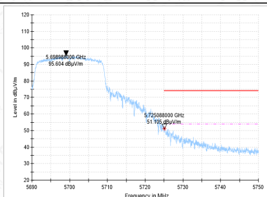
BANDEGE-11N-CH140-AV
