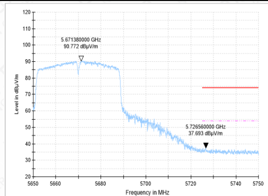
BANDEGE-11AC(40M)-CH134-AV
