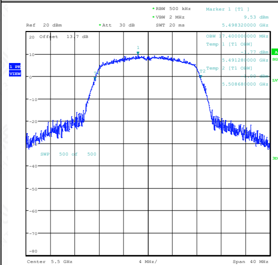
11A-Ant1-5500
