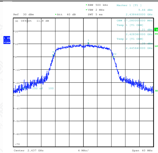
11G-Ant1-2437
