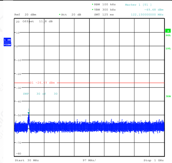
11G-Ant1-2437-30~1000-PASS
