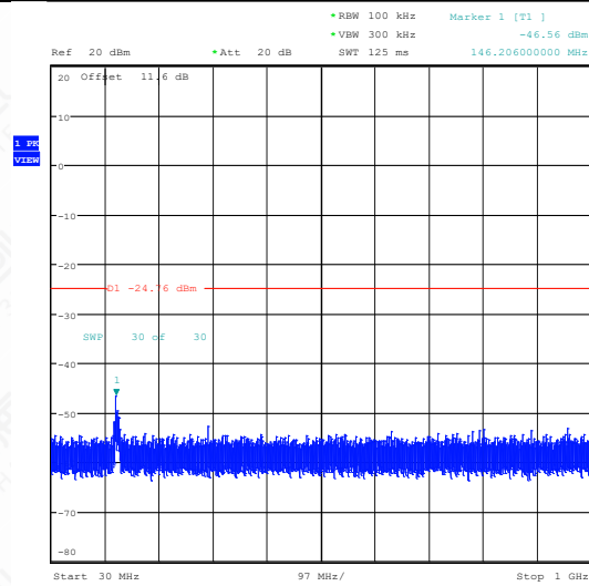
11G-Ant1-2462-30~1000-PASS
