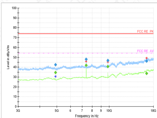
RSE-11B-CH11-3GHz-18GHz
