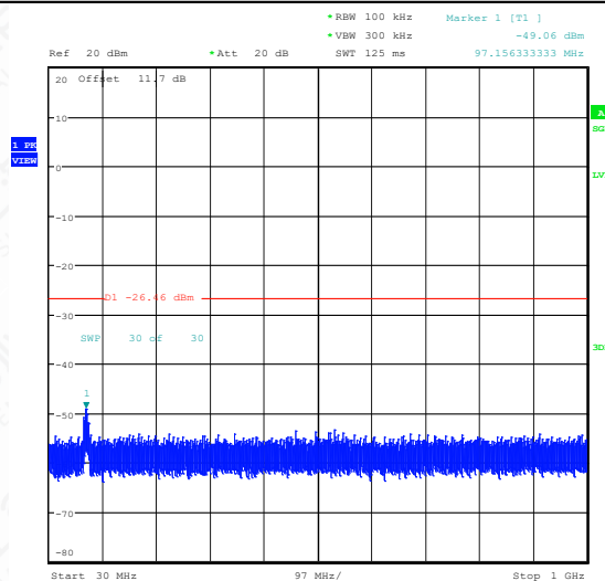
11G-Ant1-2412-30~1000-PASS
