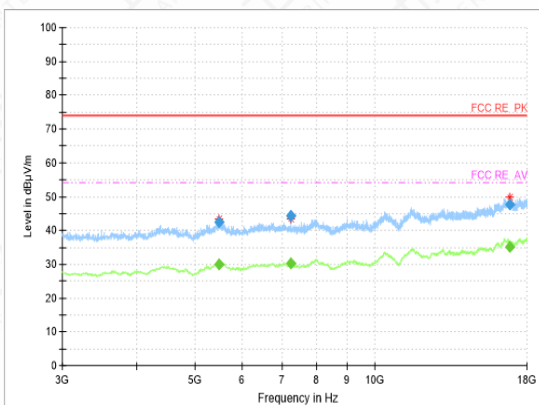
RSE-11G-CH6-3GHz-18GHz
