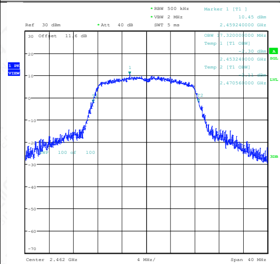
11G-Ant1-2462
