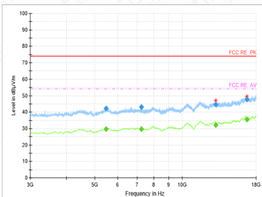
RSE-11N-CH1-3GHz-18GHz
