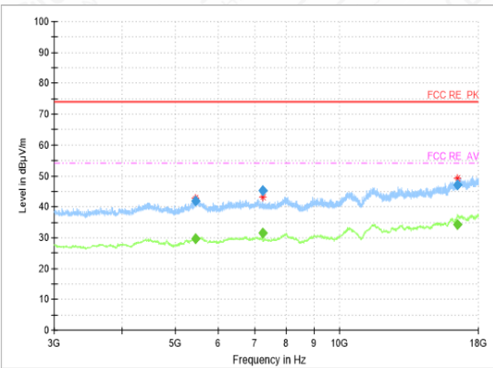
RSE-11G-CH1-3GHz-18GHz
