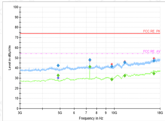
RSE-11B-CH6-3GHz-18GHz
