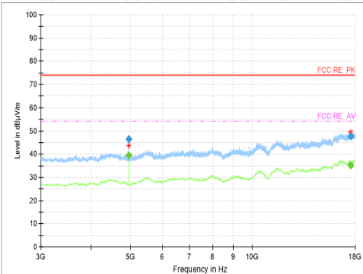
RSE-DH5-CH78-3GHz-18GHz
