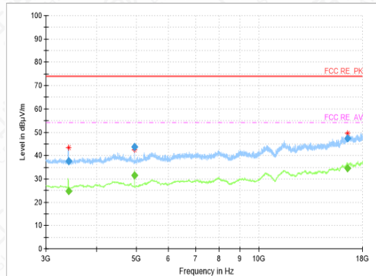
RSE-2DH5-CH78-3GHz-18GHz
