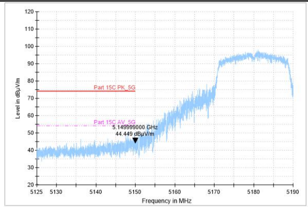
AV detector
