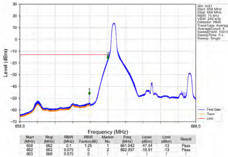
Band71_5MHz_16QAM_LCH_665.5MHz_RB_1_0_NTNV
