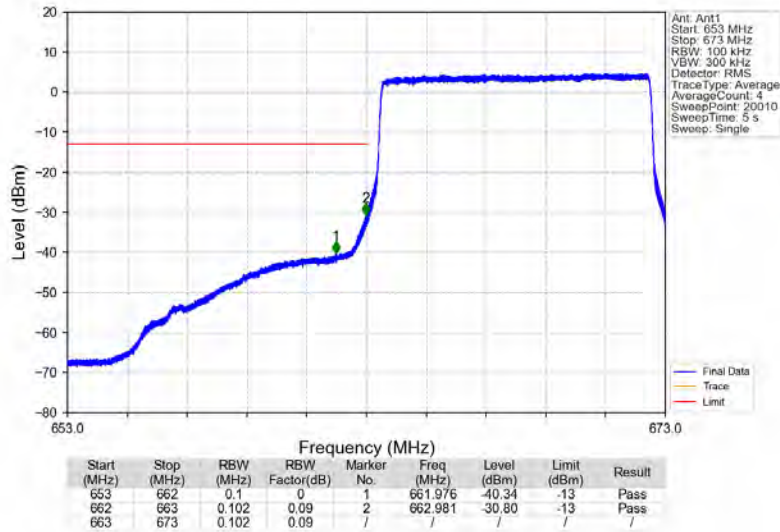
Band71_10MHz_QPSK_LCH_668MHz_RB_50_0_NTNV
