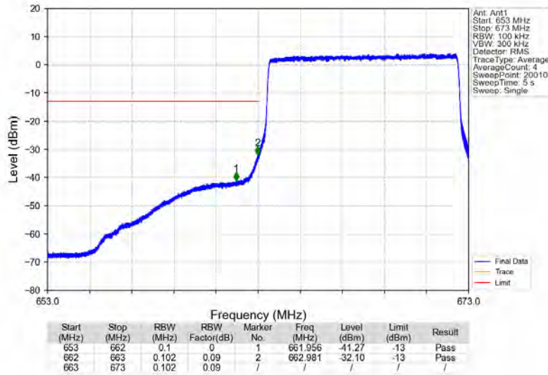
Band71_10MHz_16QAM_LCH_668MHz_RB_50_0_NTNV
