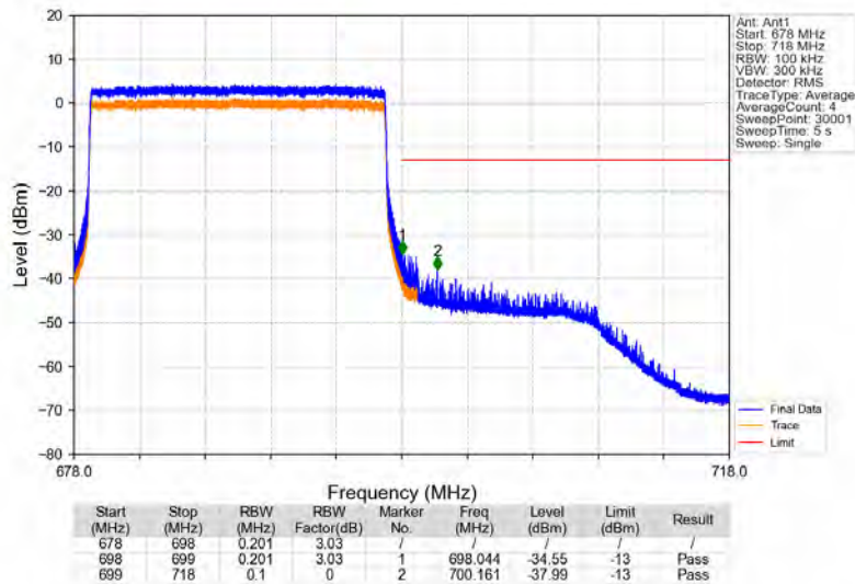
Band71_20MHz_16QAM_HCH_688MHz_RB_100_0_NTNV
