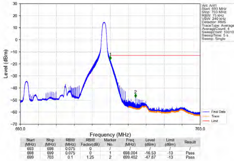
Band71_5MHz_QPSK_HCH_695.5MHz_RB_1_24_NTNV
