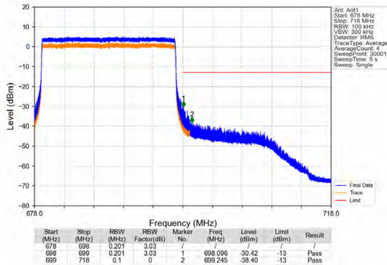
Band71_20MHz_QPSK_HCH_688MHz_RB_100_0_NTV
