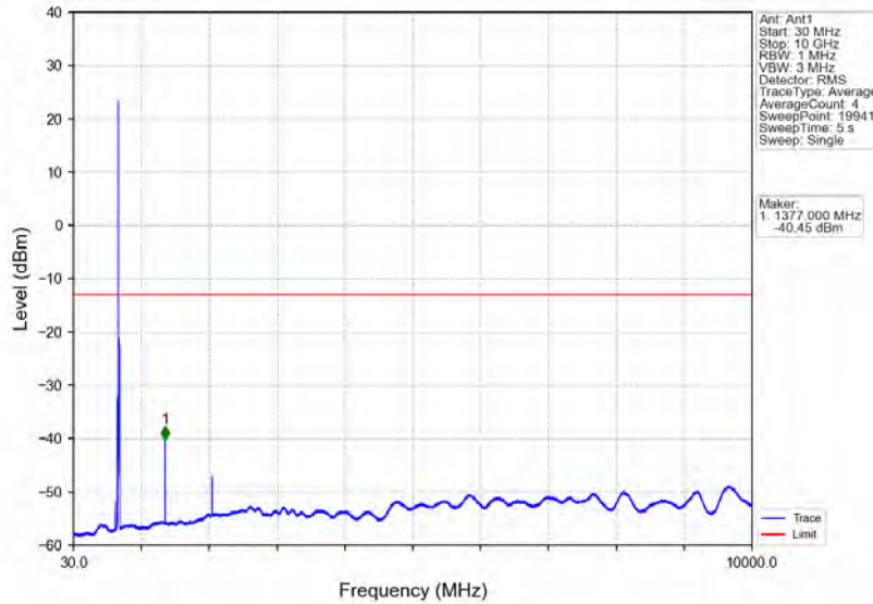
Band71_10MHz_QPSK_HCH_693MHz_RB_1_49_NTNV
