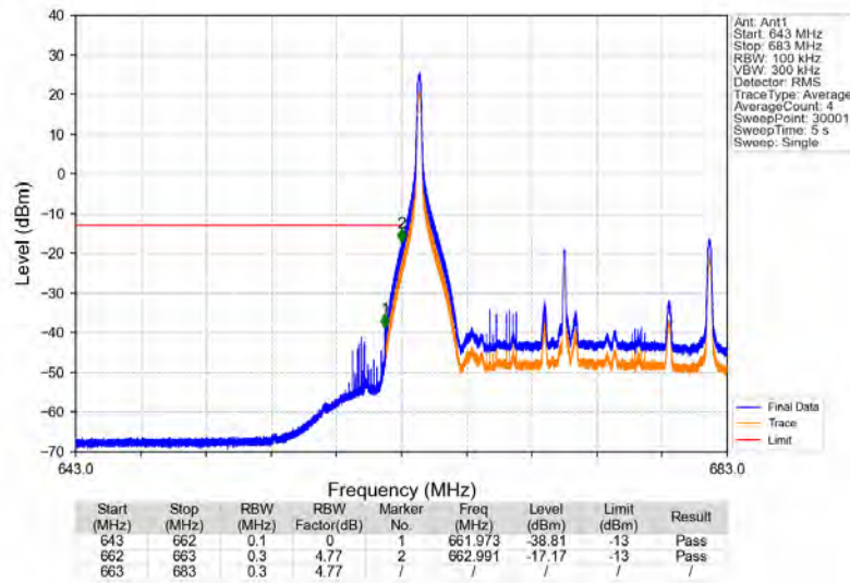
Band71_20MHz_16QAM_LCH_673MHz_RB_1_0_NTV
