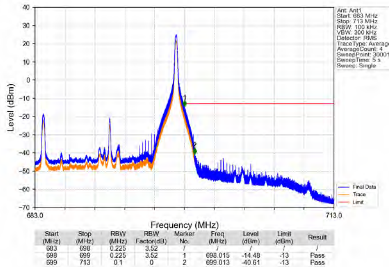
Band71_15MHz_QPSK_HCH_690.5MHz_RB_1_74_NTNV
