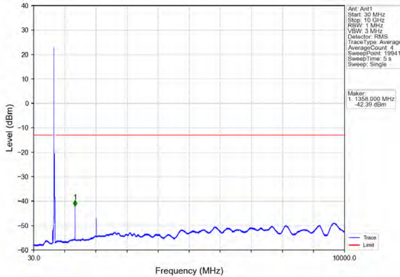
Band71_20MHz_QPSK_HCH_688MHz_RB_1_99_NTNV
