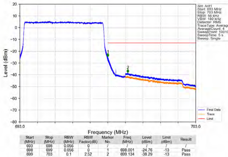
Band71_5MHz_QPSK_HCH_695.5MHz_RB_25_0_NTNV
