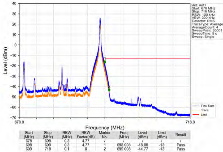
Band71_20MHz_QPSK_HCH_688MHz_RB_1_99_NTNV
