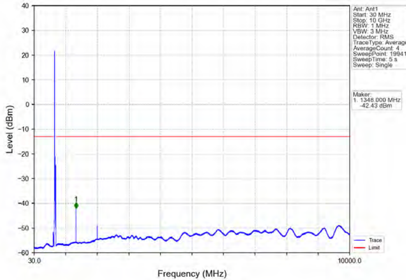
Band71_20MHz_16QAM_HCH_688MHz_RB_1_0_NTNV
