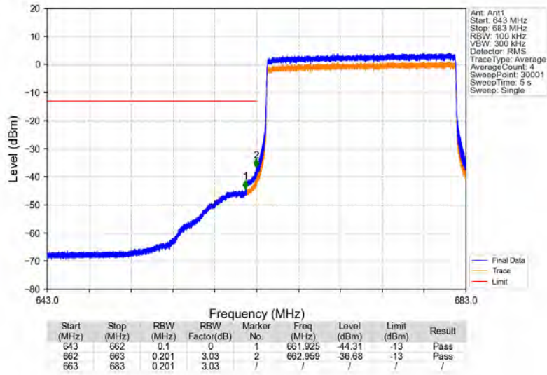
Band71_20MHz_16QAM_LCH_673MHz_RB_100_0_NTNV
