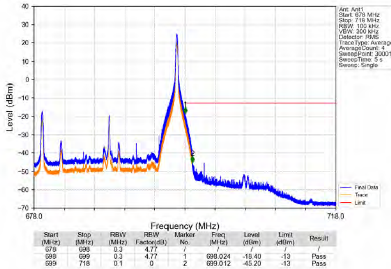
Band71_20MHz_64QAM_HCH_688MHz_RB_1_99_NTNV
