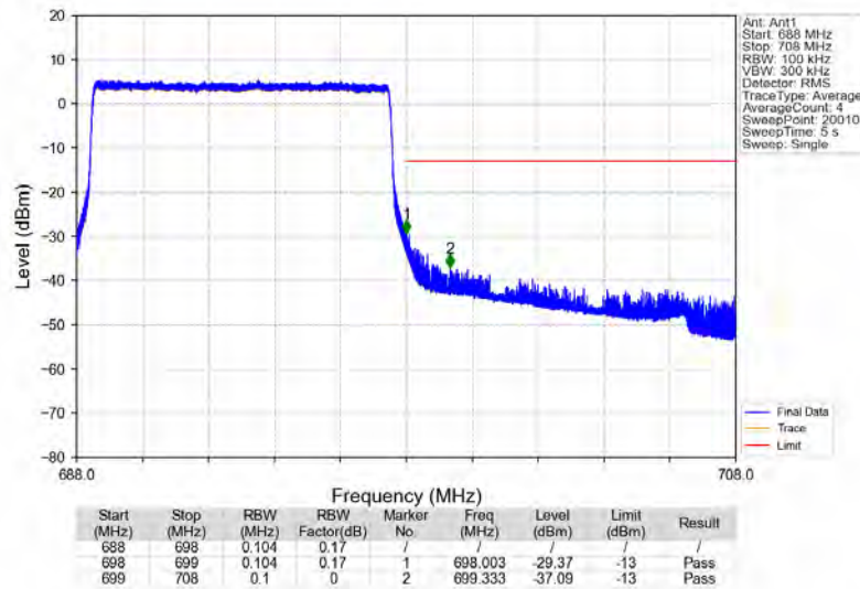
Band71_10MHz_QPSK_HCH_693MHz_RB_50_0_NTNV
