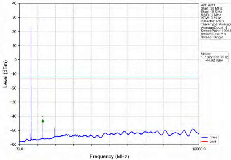
Band71_10MHz_16QAM_LCH_668MHz_RB_50_0_NTNV
