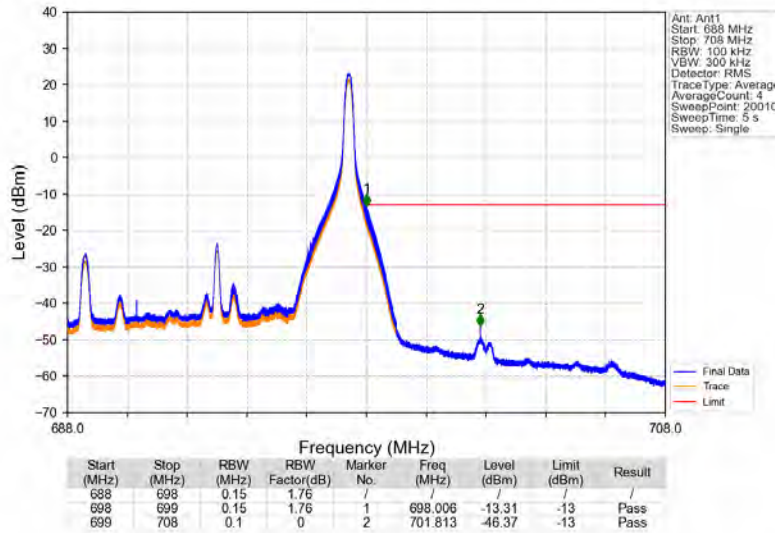
Band71_10MHz_QPSK_HCH_693MHz_RB_1_49_NTNV
