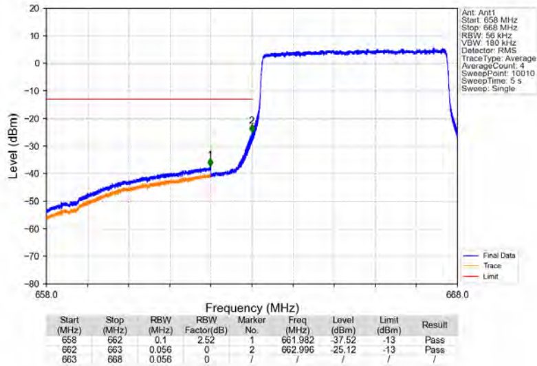
Band71_5MHz_QPSK_LCH_665.5MHz_RB_25_0_NTNV
