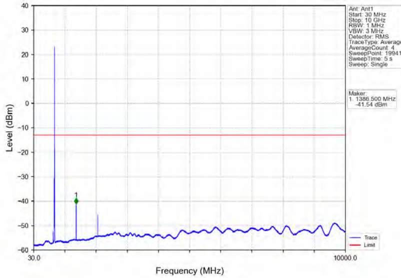
Band71_5MHz_QPSK_HCH_695.5MHz_RB_1_24_NTNV
