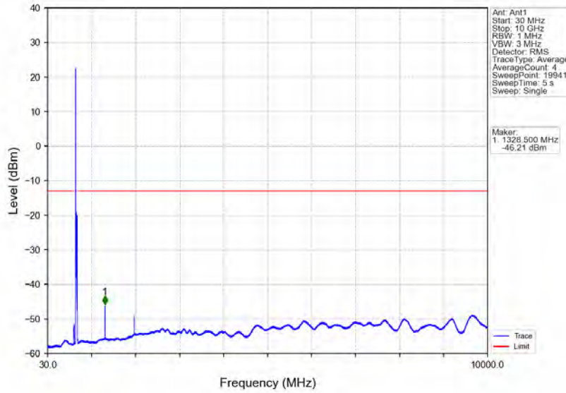
Band71_20MHz_16QAM_LCH_673MHz_RB_100_0_NTNV
