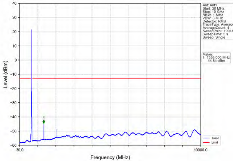
Band71_20MHz_64QAM_HCH_688MHz_RB_1_99_NTNV
