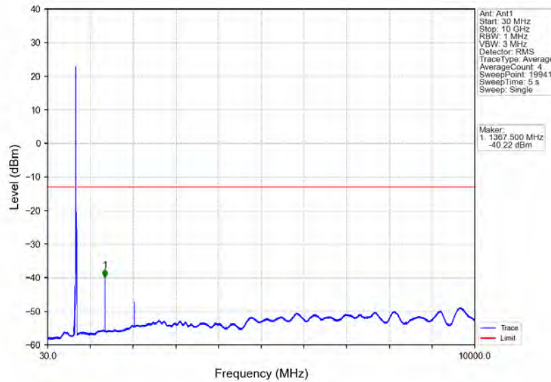
Band71_15MHz_QPSK_HCH_690.5MHz_RB_1_74_NTNV
