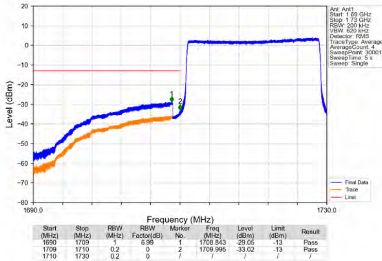
Band66_20MHz_QPSK_LCH_1720MHz_RB_100_0_NTNV
