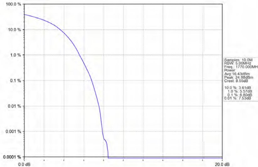
Band66_20MHz_QPSK_HCH_1770MHz_RB_100_0_NTNV
