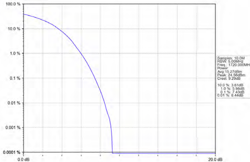
Band66_20MHz_16QAM_LCH_1720MHz_RB_100_0_NTNV
