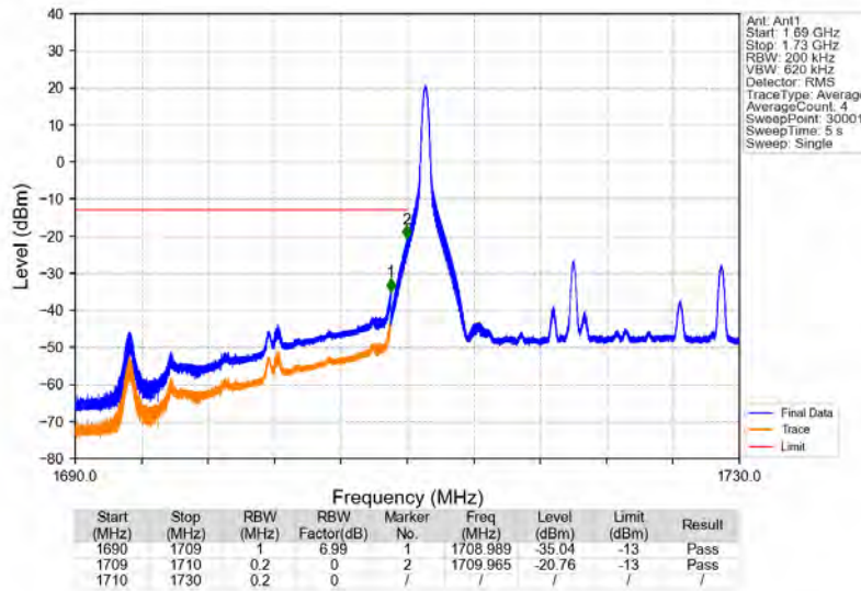
Band66_20MHz_16QAM_LCH_1720MHz_RB_1_0_NTNV
