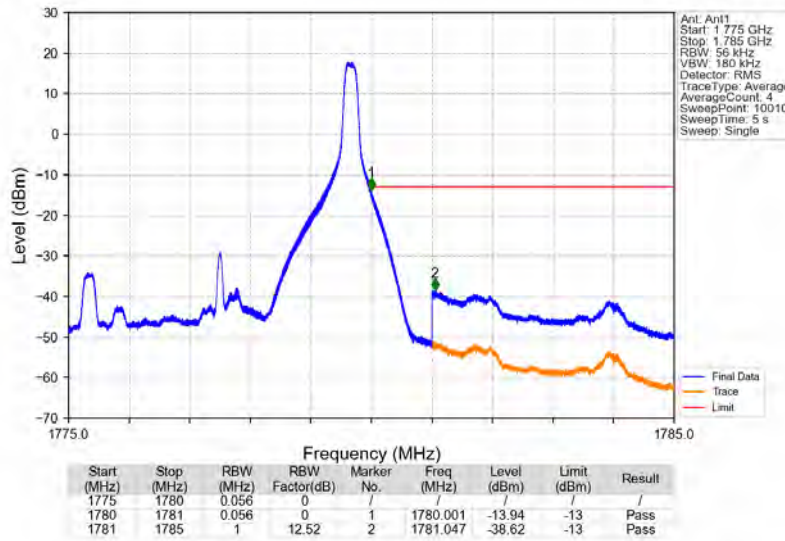
Band66_5MHz_QPSK_HCH_1777.5MHz_RB_1_24_NTNV
