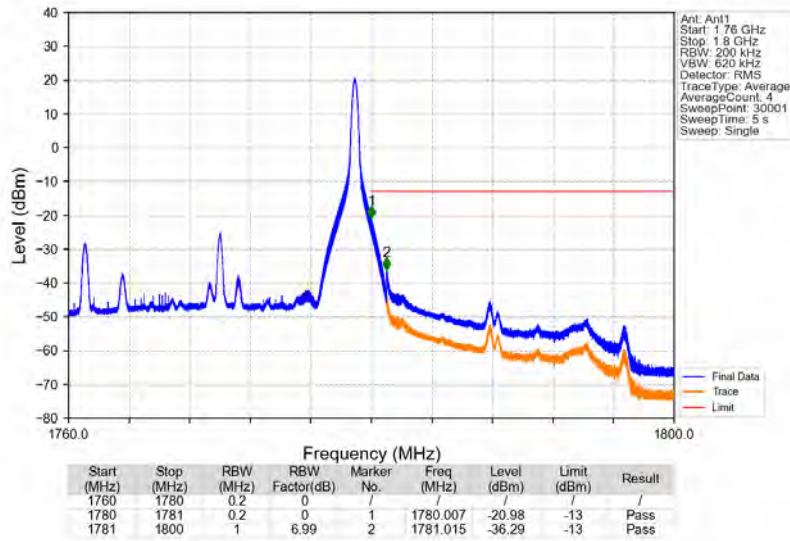
Band66_20MHz_16QAM_HCH_1770MHz_RB_1_99_NTNV
