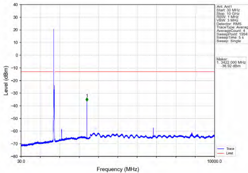
Band66_20MHz_16QAM_LCH_1720MHz_RB_1_0_NTNV
